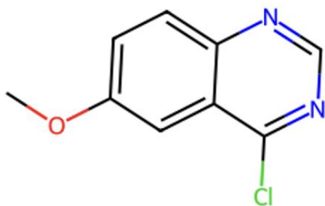
Молекул А
