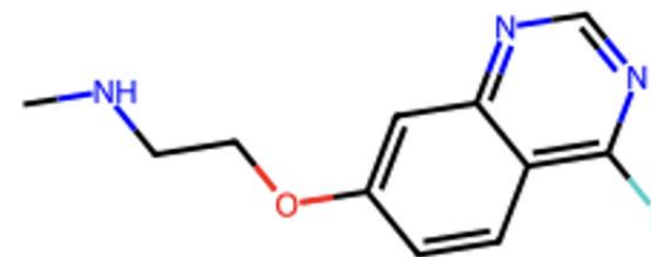
Молекул Б
